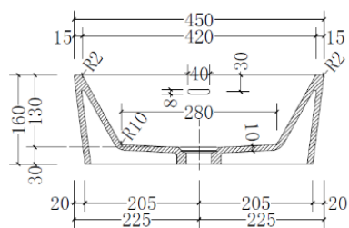
A-A Section
