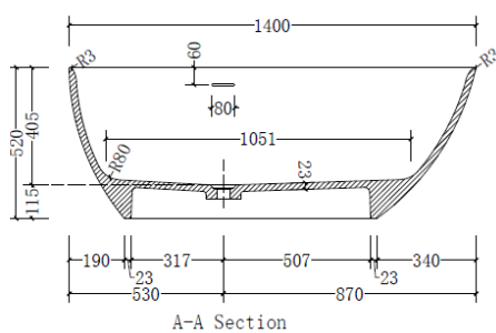
A-A Section
