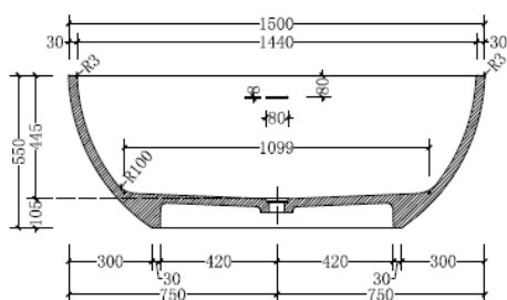
A-A Section
