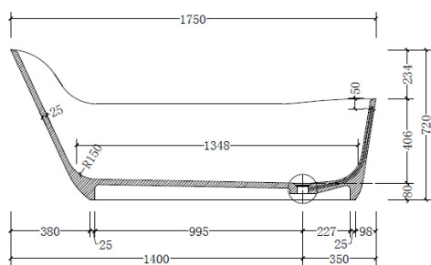
A-A Section
