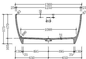
A-A Section
